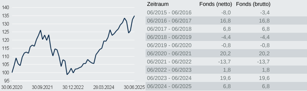
Wertentwicklung (in %) - Anteilsklasse LD
